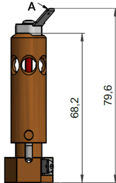
R-AMFE dimensions
